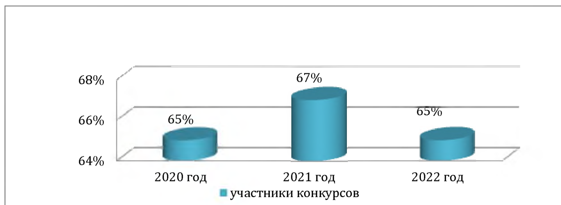
Диаграмма 12.
